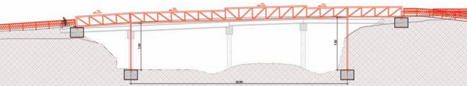
TRAM PONT METAL·LIC FERROCARRIL E: 1/200
